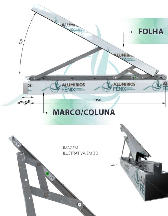
Braços projetantes CX17 Aplicação Maxim-ar Fachadas
