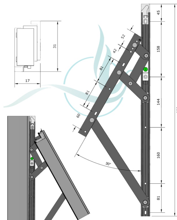
Braços projetantes CX17 Aplicação Maxim-ar Fachadas
