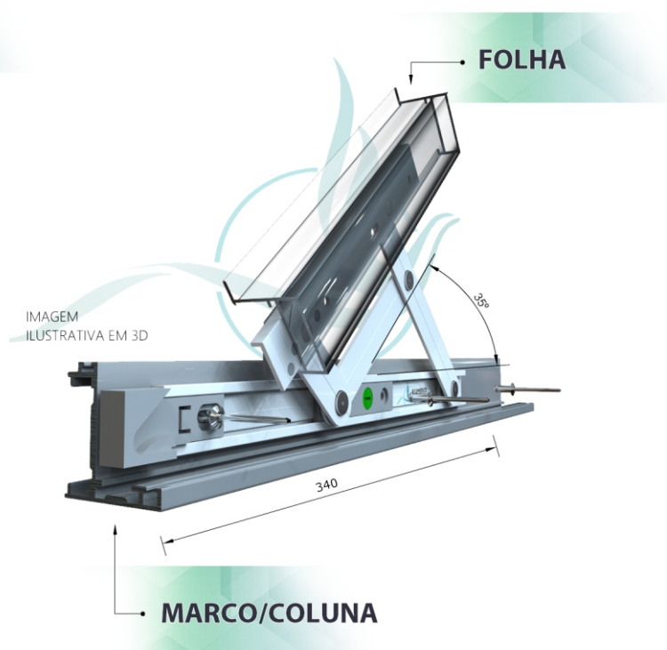
Braços projetantes CX17 Aplicação Maxim-ar Fachadas
